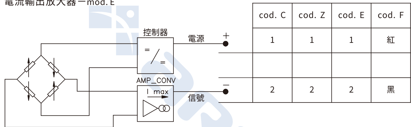
電流輸出放大器—mod. E
