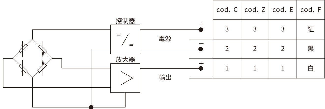
電壓輸出放大器
